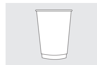
14 OZ 430ml 中空杯 规格: \phi :89 H:126 \phi :60 装箱数: 25只 20条
