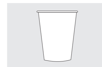
12 OZ 380ml 单层纸杯 规格: \phi :89 H:111 \phi :58 装箱数: 50只 20条
