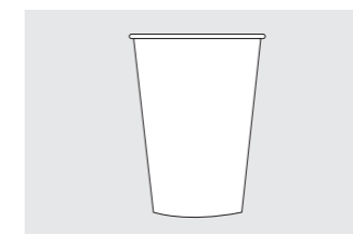
14 OZ 430ml 单层纸杯 规格: \phi :89 H:126 \phi :60 装箱数: 50只 20条
